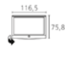
Настенный вариант Глубина телевизора: 9,5 Общая глубина: 10,9 Wall Mount Flex 52 L Общая глубина: макс. 61,6
